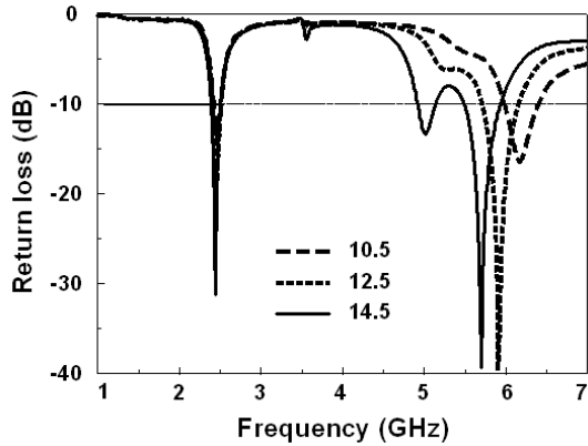
그림 2. 작은 Y-슬롯 세로 길이 변화에 따른 반사 손실 Fig. 2. Variation of return loss with the length of small Y-slot.
