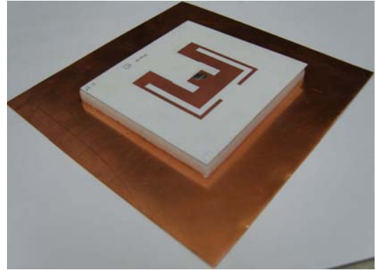
그림 7. 구현된 두 개의 Y-슬롯을 가지는 마이크로 스트립 안테나
