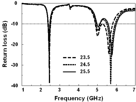
그림 6. 급전점 위치에 따른 반사 손실 Fig. 6. Variation of return loss with the feed point position.
