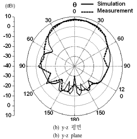
그림 10. 5.69 GHz에서의 복사 패턴 Fig. 10. Radiation patterns at 5.69 GHz.
