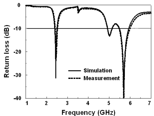
그림 8. 최적화 된 안테나의 반사 손실 Fig. 8. Return loss of the optimized antenna.
