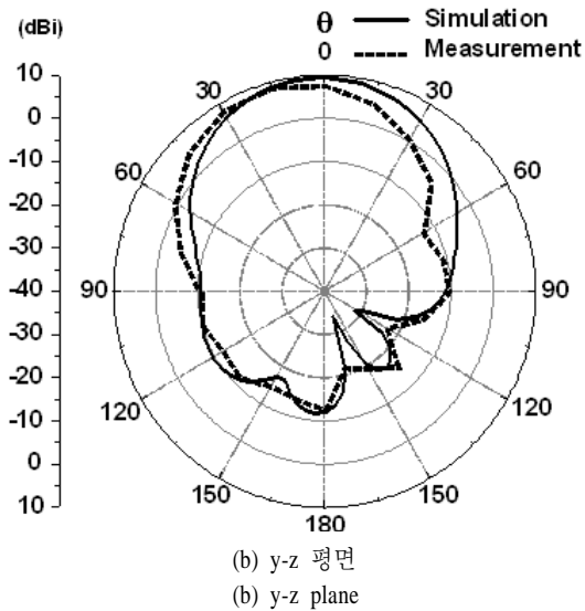
그림 9. 2.44 GHz에서의 복사 패턴 Fig. 9. Radiation patterns at 2.44 GHz.
